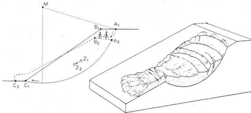
Fig. 6: Schema van een verglijding (uit 'Levende aarde in de Vlaamse Ardennen' van M-Chr. Gottigny, 1987).
