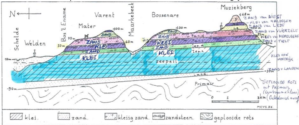
Fig. 8: Dwarsdoorsnede door het reliëf en de geologie van de Vlaamse Ardennen (M-Chr. Gottigny).
