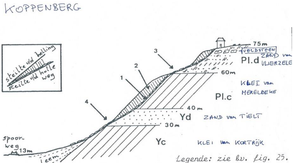
Fig. 5: het geologisch dwarsprofiel langs de holle weg van de Koppenberg te Melden (figuur uit 'Levende aarde in de Vlaamse Ardennen' van M-Chr. Gottigny, 1987).
